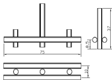
CRUZETA TUBULAR
